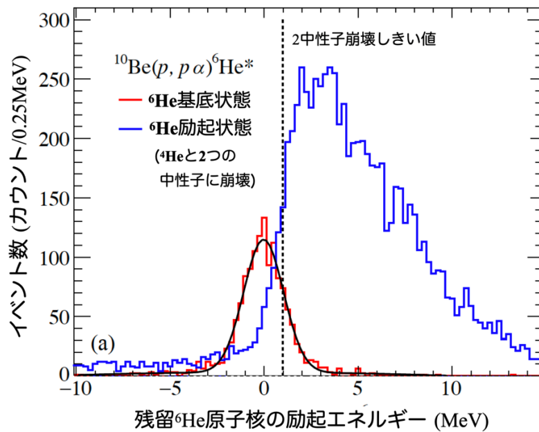
図2 ノックアウト反応後に生じた {}^6\text{He} 原子核の励起エネルギースペクトル
